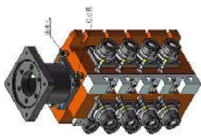
ER 4+4+J4 动力头 ER 4+4+J4 Power Head
